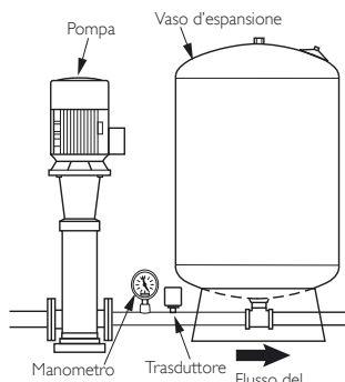
Fig. 1.4-6 Installazione su gruppo aumento pressione con vaso
