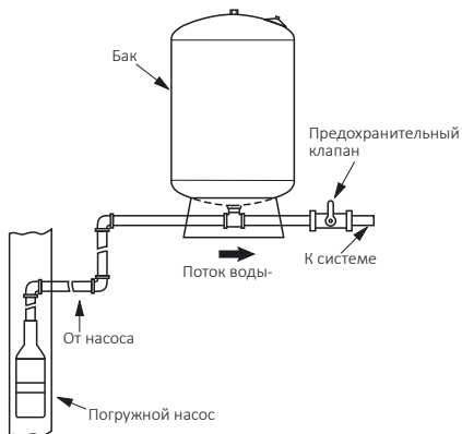
Рис. 1.4-3 С погружным насосом
